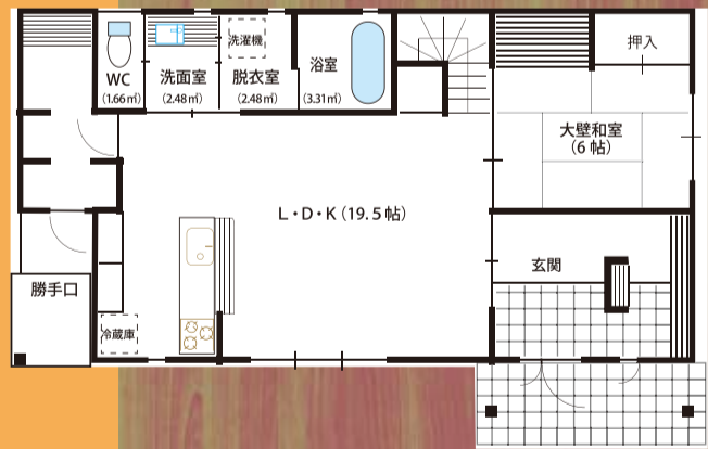
1階平面図
