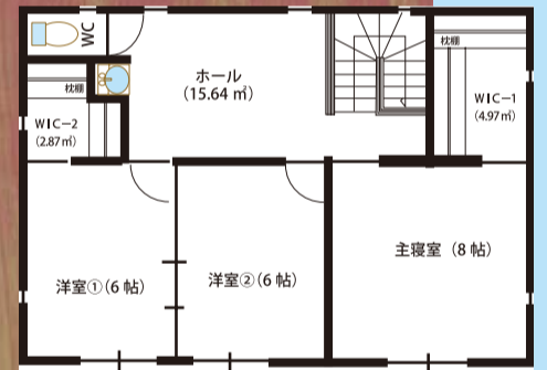
2階平面図
