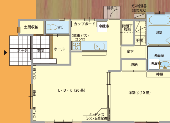
1階平面図
